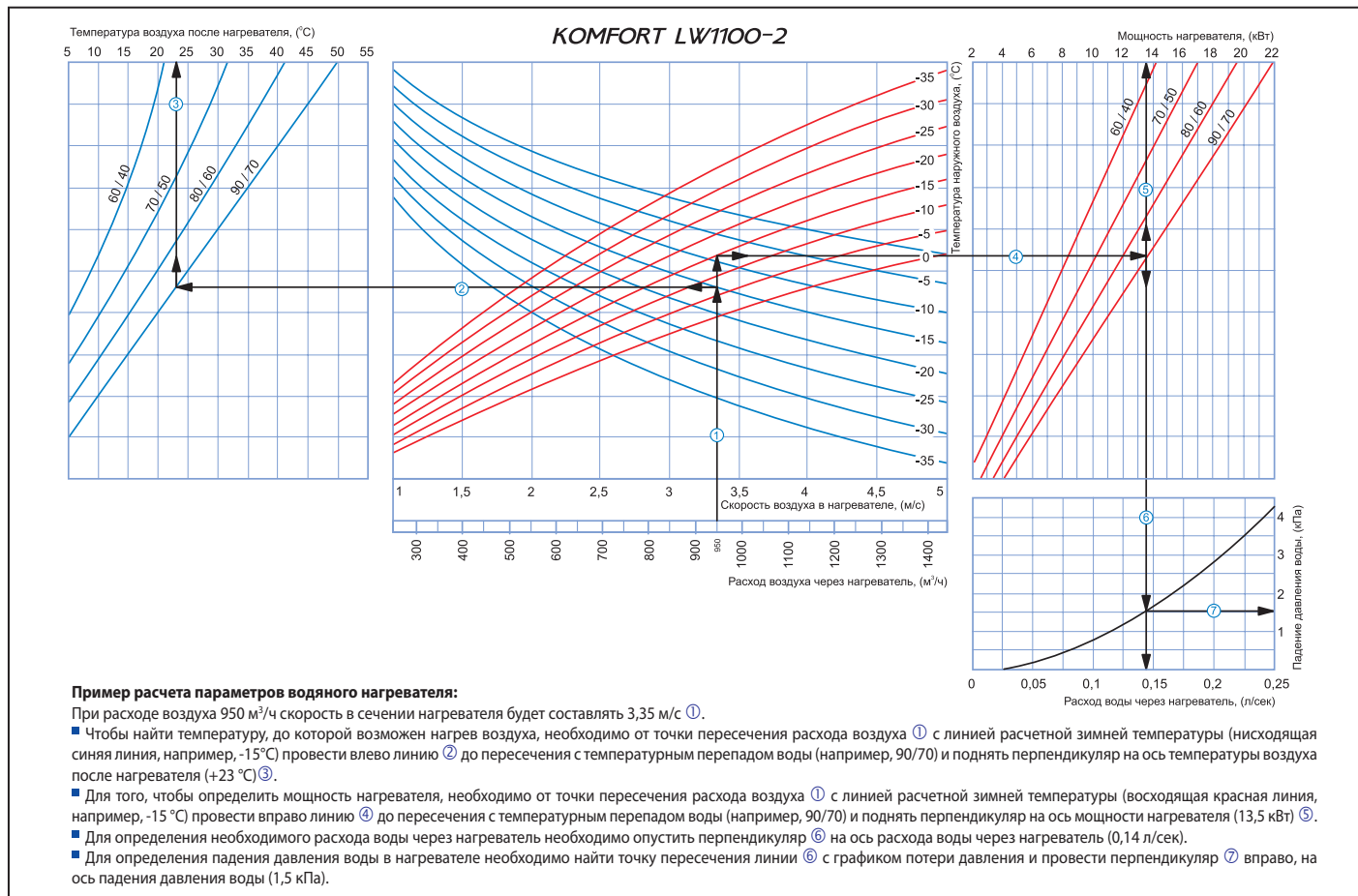
Рис. 6. Расчет водяного нагревателя KOMFORT LW1100-2
