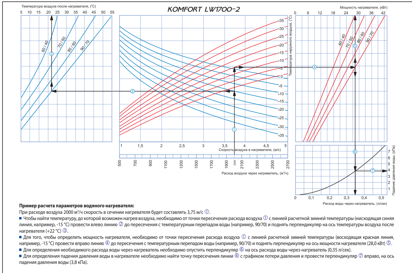
Рис. 8. Расчет водяного нагревателя KOMFORT LW1700-2
