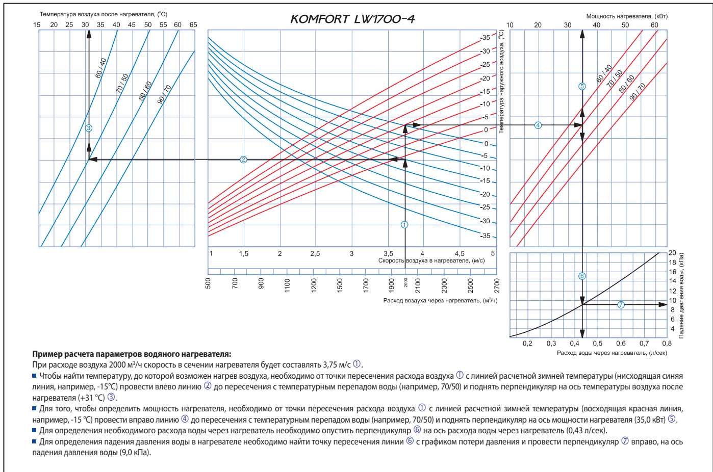
Рис. 9. Расчет водяного нагревателя KOMFORT LW1700-4
