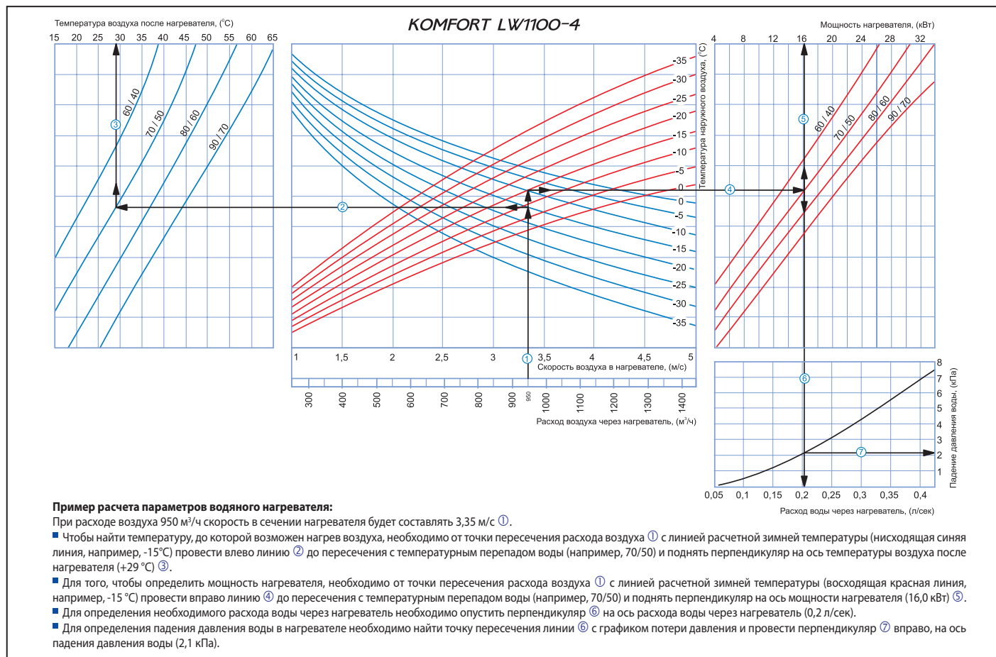
Рис. 7. Расчет водяного нагревателя KOMFORT LW1100-4
