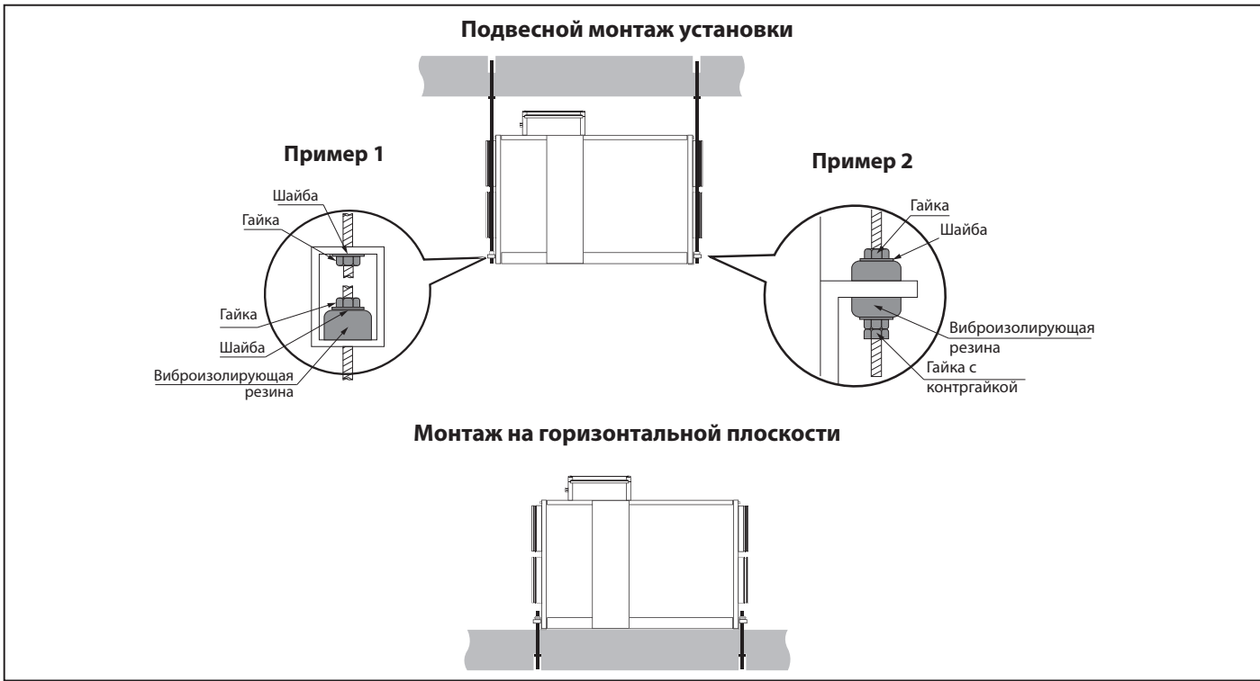
Рис. 13. Монтаж
