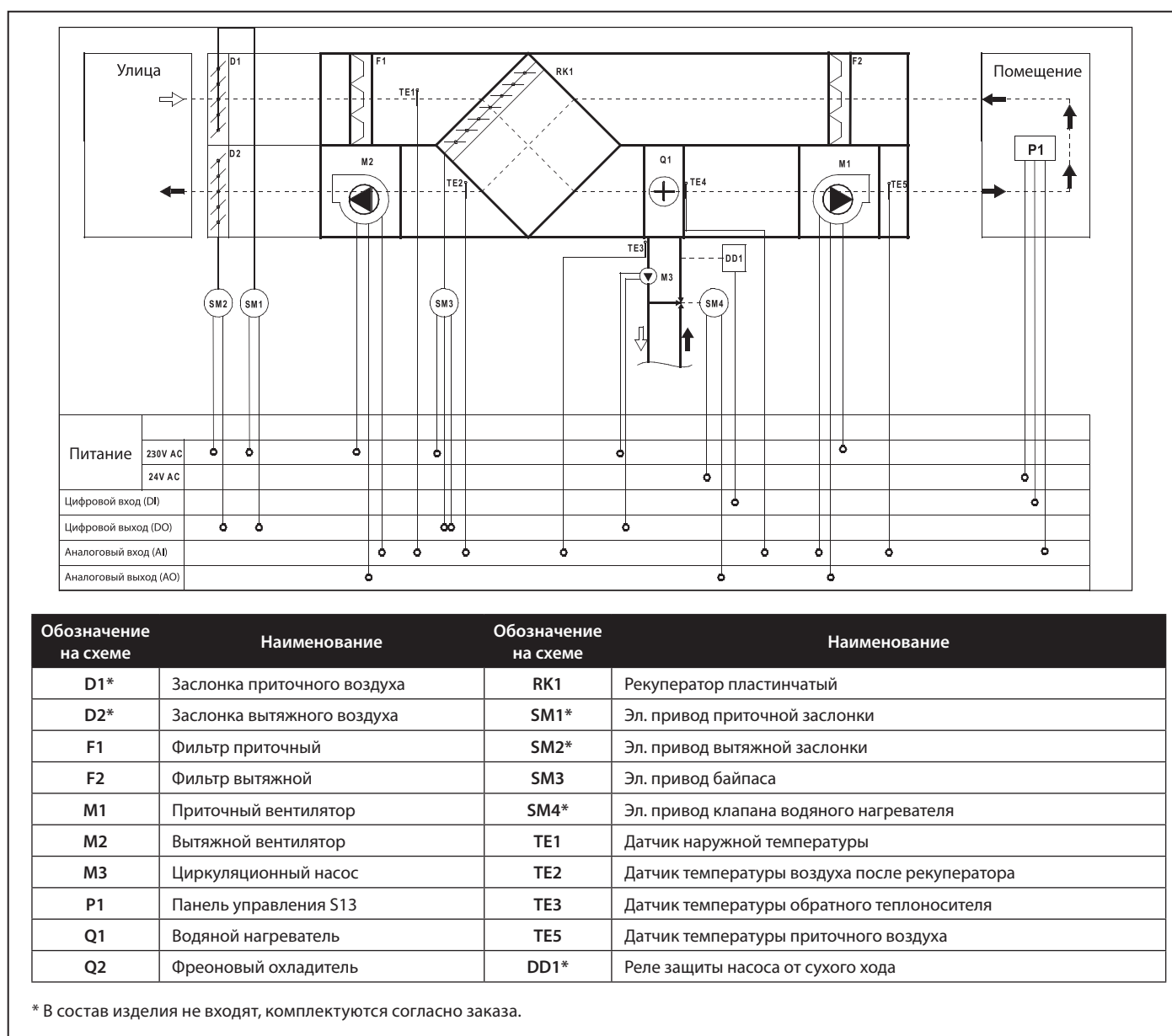
Рис. 19. Функциональная схема
