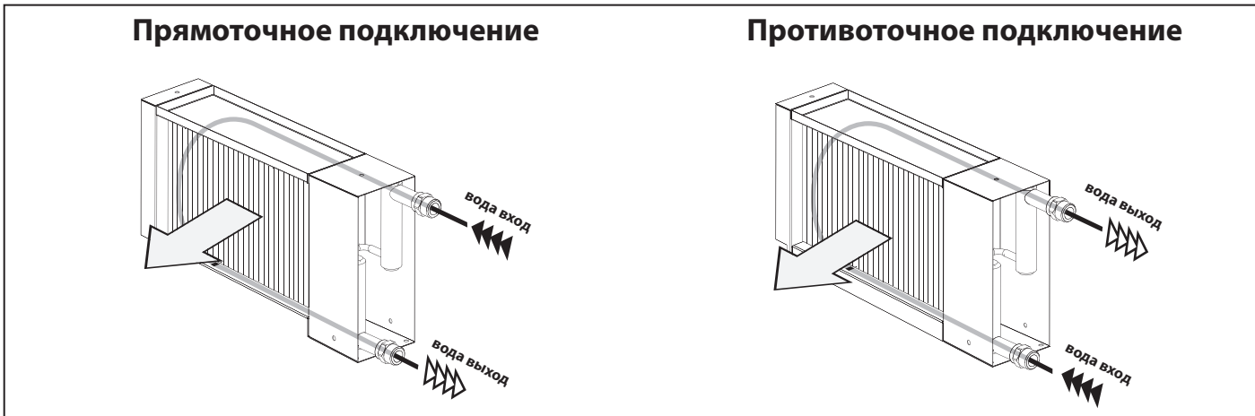
Рис. 14. Подключение водяного нагревателя
