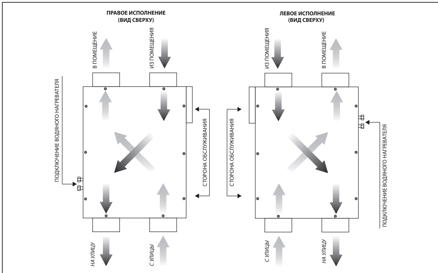
Рис. 2. Исполнение установок KOMFORT EC DW600-2 / DW1000-4
