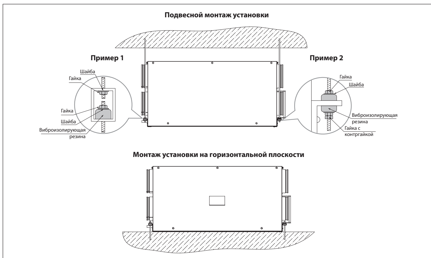
Рис. 6. Монтаж
