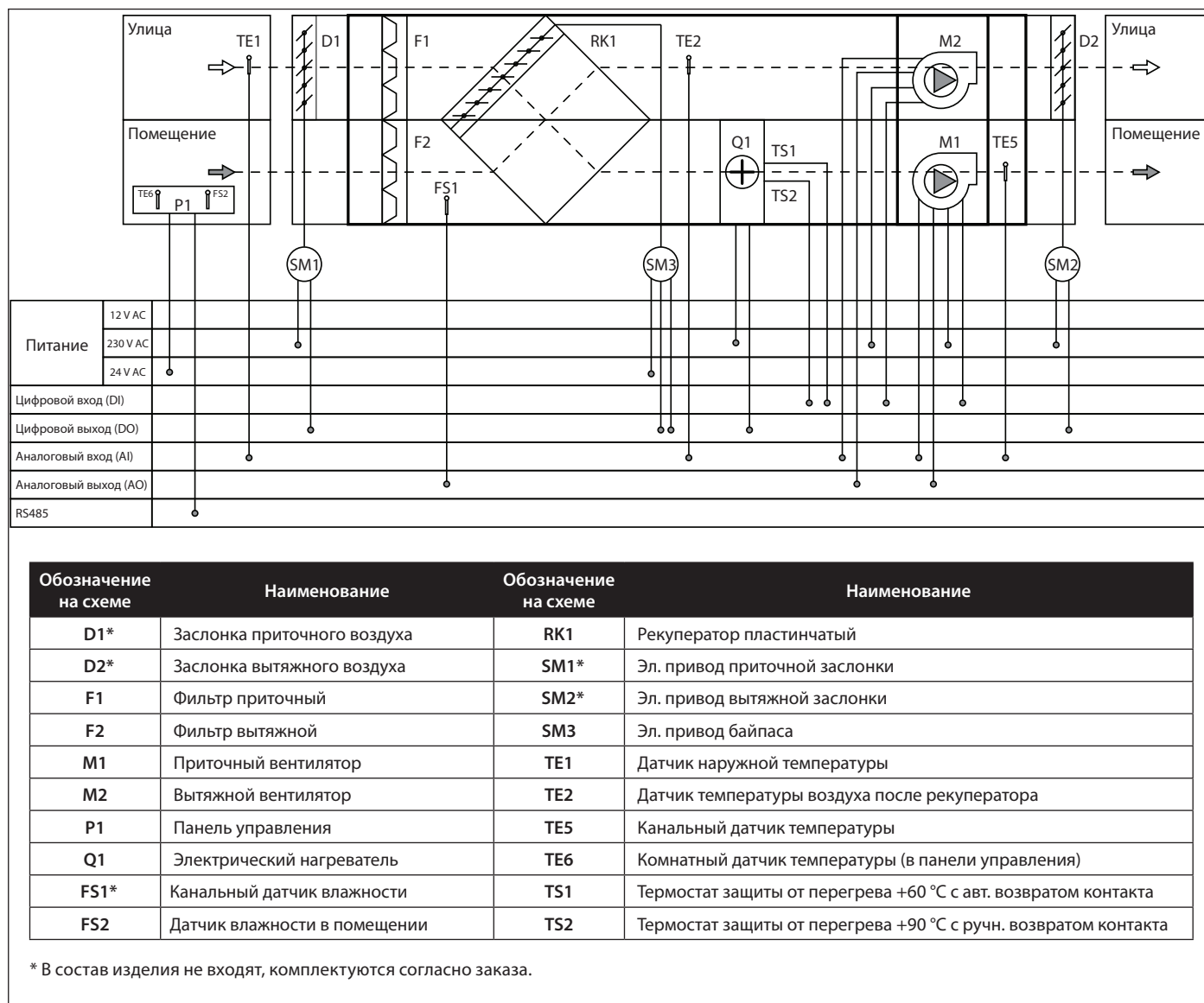
Рис. 12. Функциональная схема KOMFORT EC DE2000-12 ... EC DE4000-21
