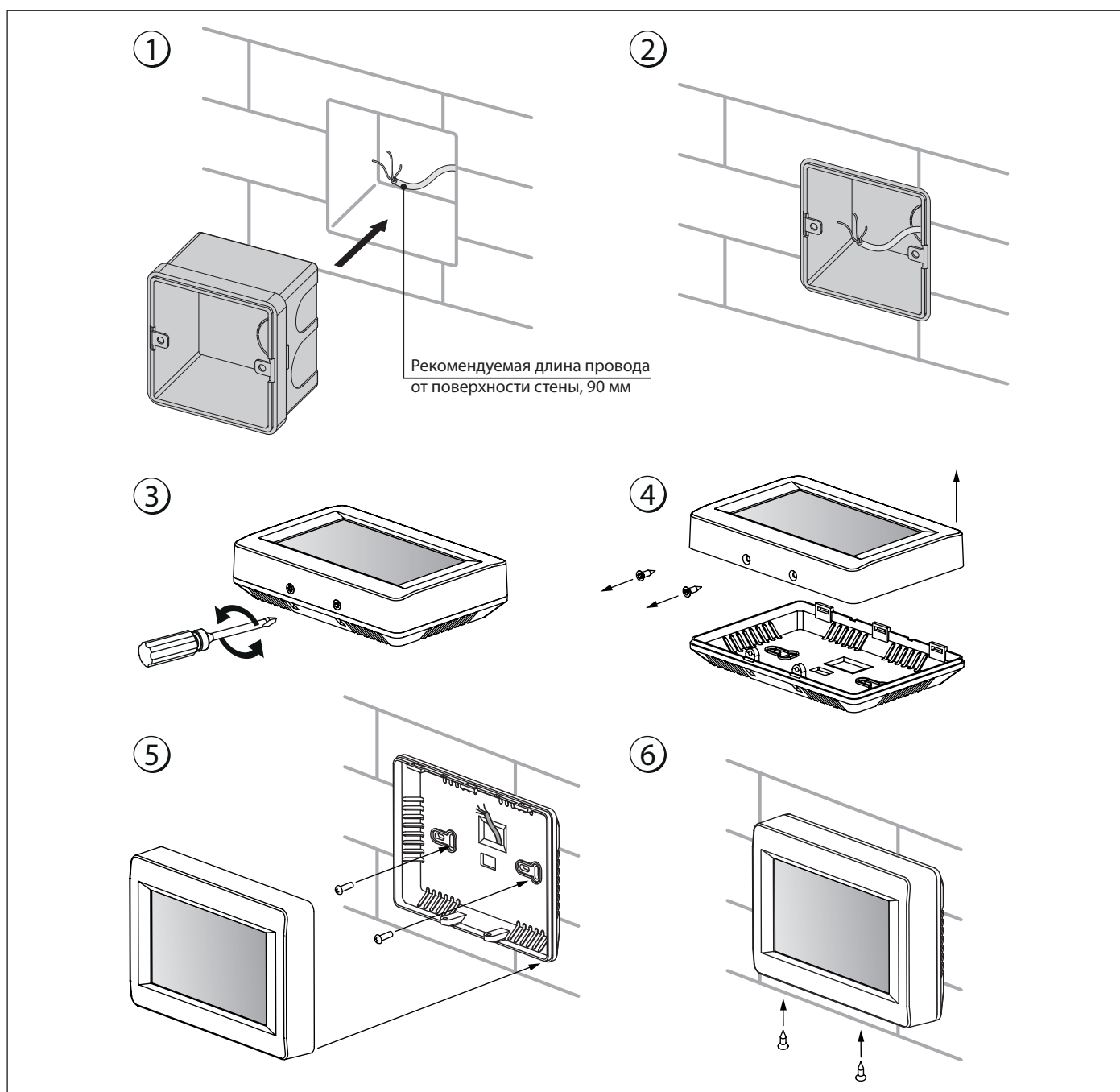
Рис. 15. Монтаж панели управления
