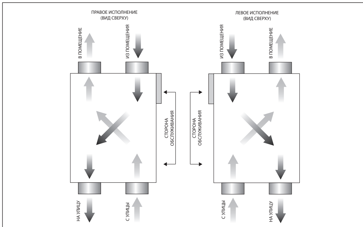
Рис. 2. Исполнение установок KOMFORT EC DE400/700/1100
