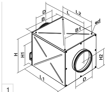
Габаритные и присоединительные размеры вентилятора Iso-ZS с одним входным и одним выходным патрубком
